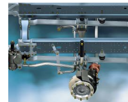
Однолистовая рессора, позволяющая выиграть в весовых характеристиках
